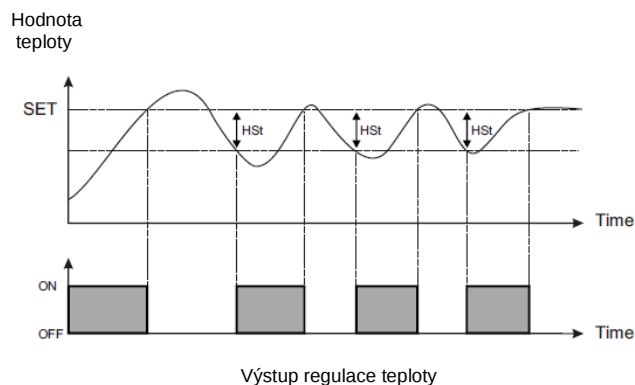
Výstup regulace teploty
